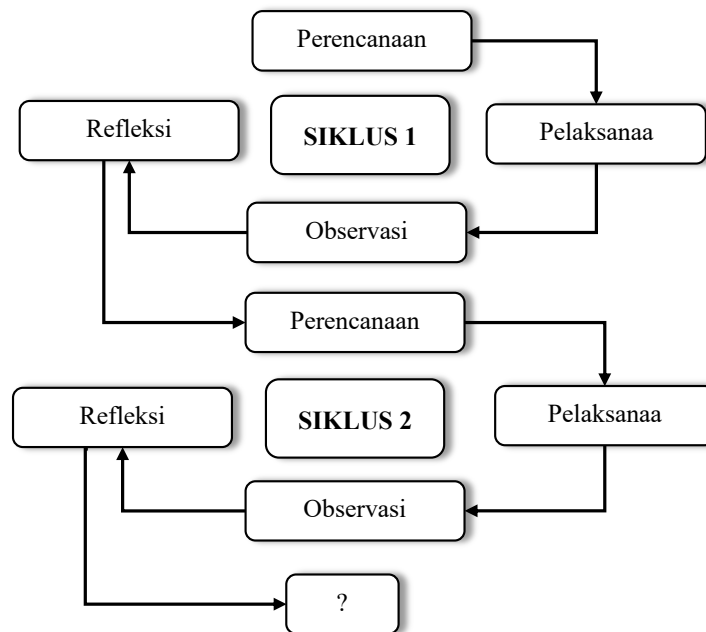
Gambar 1 Siklus Penelitian
